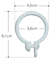
▶RN100 リングランナー 組 成：ポリプロピレン樹脂 出荷単位：100個
