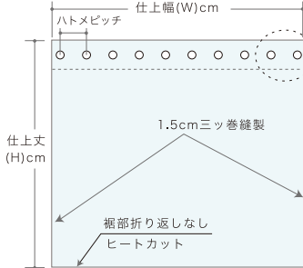
プラスチックハトメ加工 内径1.2cm 外径2.4cm
