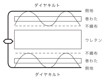
【断面図】
